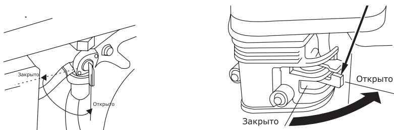
Рис. 14. Топливный кран
